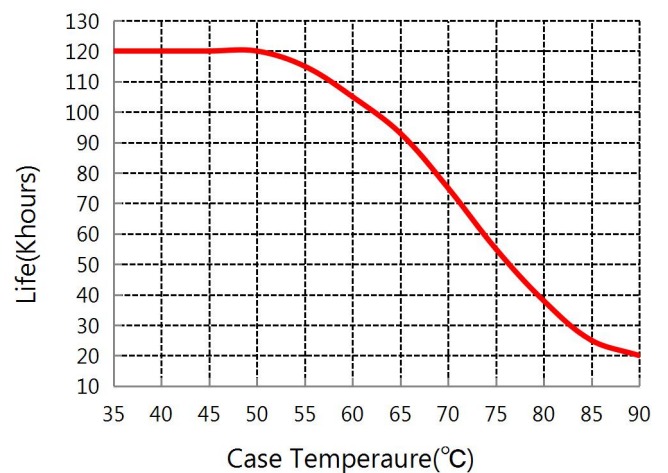
图 6 寿命-壳温曲线
